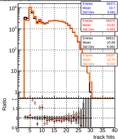
mean hit DOM_mkFit1 TTbase DOM_mkFit5 TT_retrainOldFiles125_v2_prelimWP_epoch4 DOM_mkFit6 TT_baseline_6iter DOM_mkFit6 TT_retrainOldFiles125_v2_prelimWP_epoch2_wsQCD
