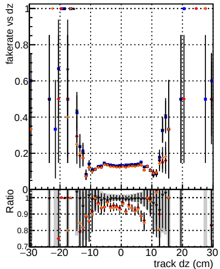
Fake rate vs dz DGM mKF15 TTbase DGM mKF15 TTbase DGM mKF16 TTbase DGM mKF16 TTbase
