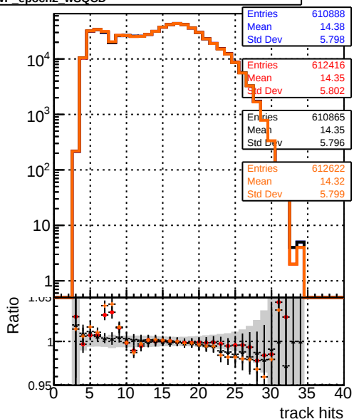
DQM_mkFit_TTbase DQM_mkFit5_TT_retrainOldFiles125_v2_prelimWP_epoch4 DQM_mkFit6_TT_baseline_6iter DQM_mkFit6_TT_retrainOldFiles125_v2_prelimWP_epoch2_wsQCD
