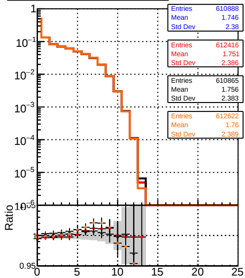
DQM_mkFit_TTbase DQM_mkFit5_TT_retrainOldFiles125_v2_prelimWP_epoch4 DQM_mkFit6_TT_baseline_6iter DQM_mkFit6_TT_retrainOldFiles125_v2_prelimWP_epoch2_wsQCD
