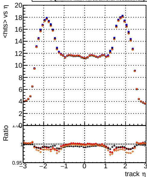
DQM_mkFit1_TTbase DQM_mkFit5_TT_retrainOldFiles125_v2_prelimWP_epoch4 DQM_mkFit6_TT_retrainOldFiles125_v2_prelimWP_epoch2_wsQCD mean hits
