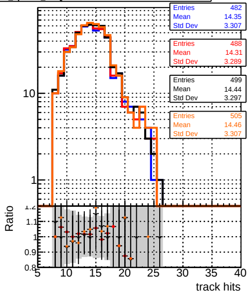
mean hit DQM_mkFit5 TTbase DQM_mkFit5 TT_retrainOldFiles125_v2_prelimWP_epoch4 DQM_mkFit6 TT_baseLine_6iter DQM_mkFit6 TT_retrainOldFiles125_v2_prelimWP_epoch2_wSQCD
