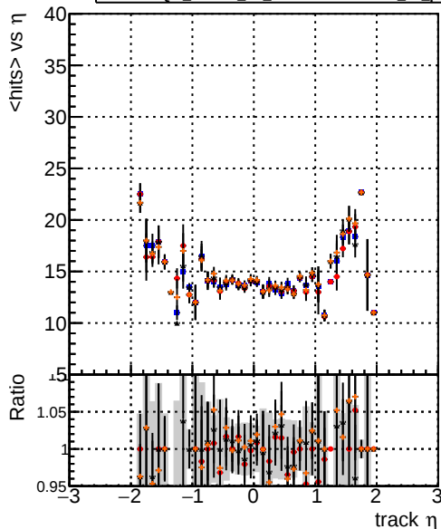
mean hit DQM_mkFit5 TTbase DQM_mkFit5 TT_retrainOldFiles125_v2_prelimWP_epoch4 DQM_mkFit6 TT_baseLine_6iter DQM_mkFit6 TT_retrainOldFiles125_v2_prelimWP_epoch2_wSQCD
