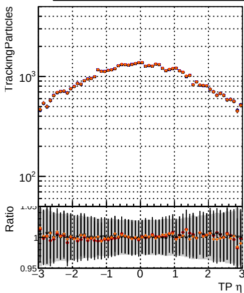
● DQM_mkFit1_TTbase ◆ DQM_mkFit5_TT_retrainOldFiles125_v2_prelimWP_epoch4 ✕ DQM_mkFit_TT_baseline_6iter ▲ DQM_mkFit6_TT_retrainOldFiles125_v2_prelimWP_epoch2_wsQCD
