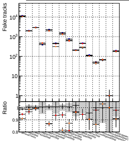
Number Model 1 DQM mkFit5 TT retrainOldFiles125 v2 prelimWP epoch4 2 DQM mkFit TT baseline 6iter 3 DQM mkFit6 TT retrainOldFiles125 v2 prelimWP epoch2 wSQCD
