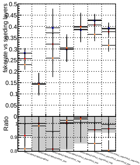
Fake rate vs. DGM mkFit TTbase DGM mkFit5 TTbase DGM mkFit6 TTbase TrainOldFiles125 v2_prelimWP_epoch4 TrainOldFiles125 v2_prelimWP_epoch2_wsQCD
