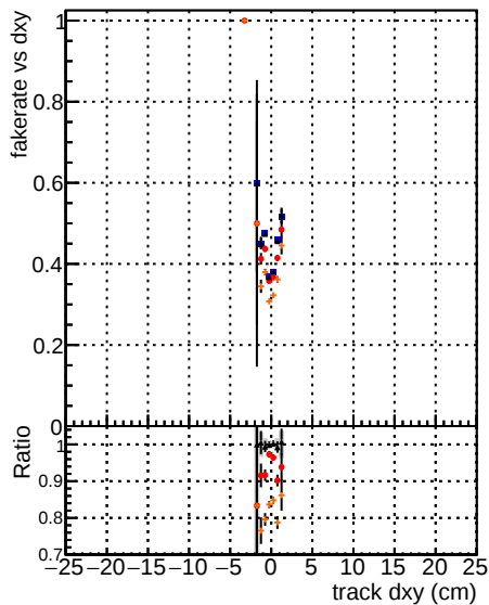
Fake rate vs d Legend: DOM PRE15 TT trainOldFiles125 v2 prelimWP epoch4 DOM PRE15 TT baselineFile DOM PRE16 TT trainOldFiles125 v2 prelimWP epoch2 wSQCD
