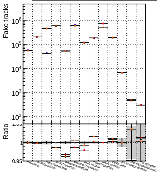
Number ● DQM mkFit5 TT retrainOldFiles125 v2 prelimWP_epoch4 ▲ DQM mkFit TT baseline 6iter ◆ DQM mkFit6 TT retrainOldFiles125 v2 prelimWP_epoch2 wSQCD ●
