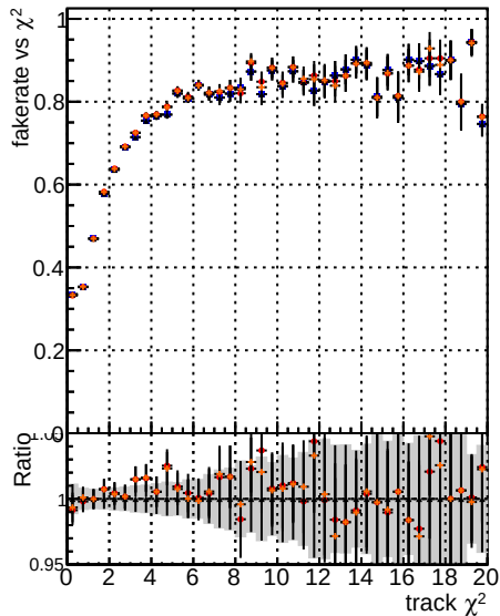
Fake rate vs. \chi^2 Legend: DQM mktFit TTbase baseLine DQM mktFit TTbase DQM mktFit TTbase DQM mktFit TTbase
