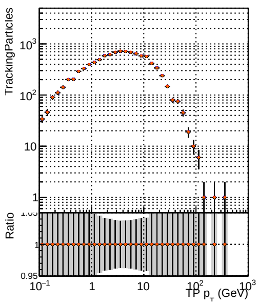
— DQM_mkFit6 TTbase — DQM_mkFit5 TT_retrainOldFiles125_v2_prelimWP_epoch4 — DQM_mkFit6 TT_baseline_6iter — DQM_mkFit6 TT_retrainOldFiles125_v2_prelimWP_epoch2_wSQCD
