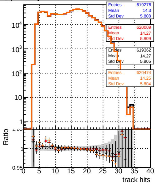
mean hits DQM_mkFit_TTbase DQM_mkFit5_TT_retrainOldFiles125_v2_prelimWP_epoch4 DQM_mkFit6_TT_retrainOldFiles125_v2_prelimWP_epoch2_wsQCD
