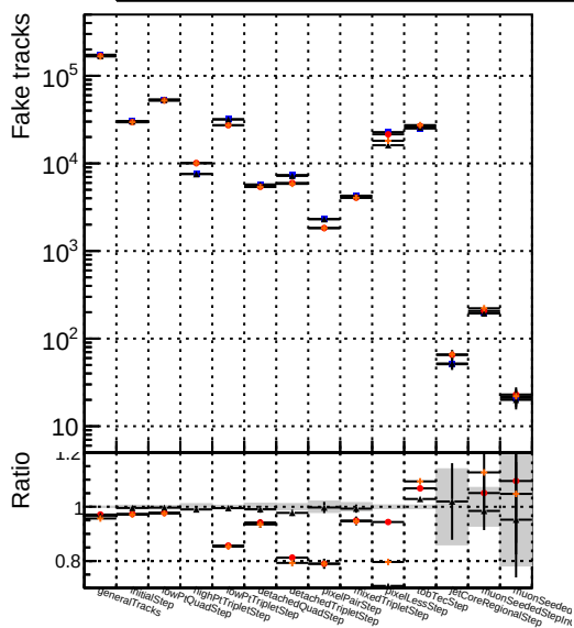
Number Model 1 DQM_mkrf15_TT_retrainOldFiles125_v2_prelimWP_epoch4 2 DQM_mkFit_TT_baseline_6iter 3 DQM_mkFit6_TT_retrainOldFiles125_v2_prelimWP_epoch4
