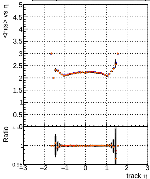
mean hits vs \eta Legend: - DQM_mkFit5_TT_base - DQM_mkFit5_TT_retrainOldFiles125_v2_prelimWP_epoch4 - DQM_mkFit6_TT_base - DQM_mkFit6_TT_retrainOldFiles125_v2_prelimWP_epoch4
