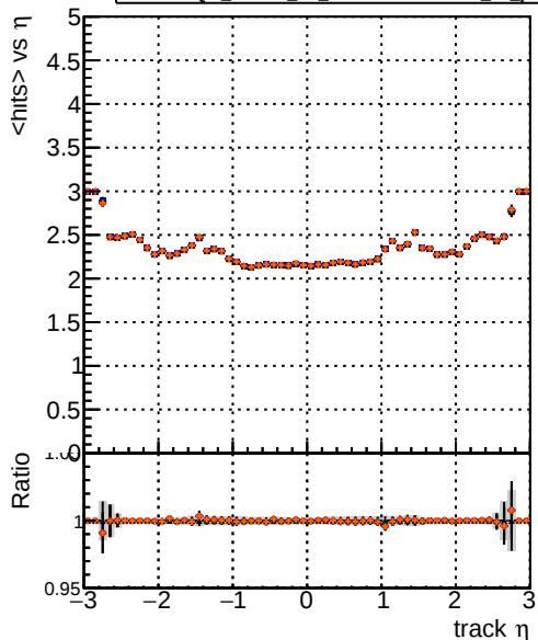
mean hit DQM_mkFit_TTbase DQM_mkFit5_TT_retrainOldFiles125_v2_prelimWP_epoch4 DQM_mkFit_TT_baseline_6iter DQM_mkFit6_TT_retrainOldFiles125_v2_prelimWP_epoch4
