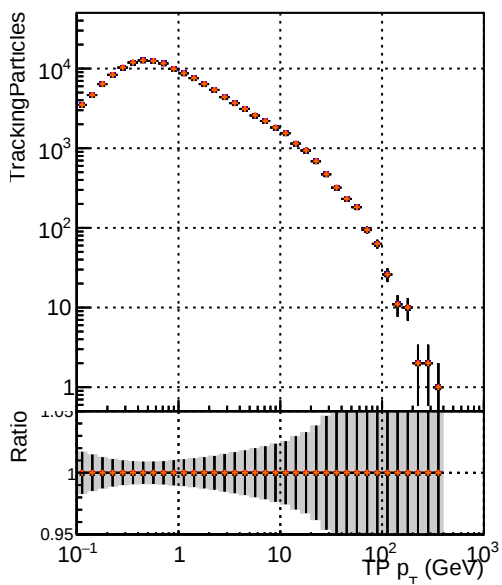
— DQM_mkFit5_TT_base — DQM_mkFit5_TT_retrainOldFiles125_v2_prelimWP_epoch4 — DQM_mkFit6_TT_base — DQM_mkFit6_TT_retrainOldFiles125_v2_prelimWP_epoch4
