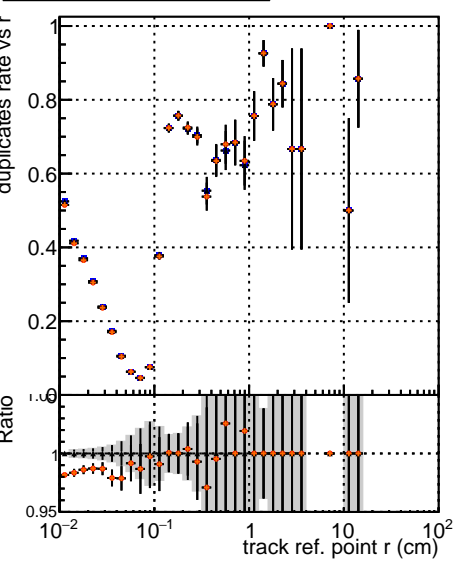
■ DQM mkFit TTbase ■ DQM mkFit5 TTbase ■ DQM mkFit6 TTbase ■ DQM mkFit5 TT_retrainOldFiles125_v2_prelimWP_epoch4 ■ DQM mkFit6 TT_retrainOldFiles125_v2_prelimWP_epoch4
