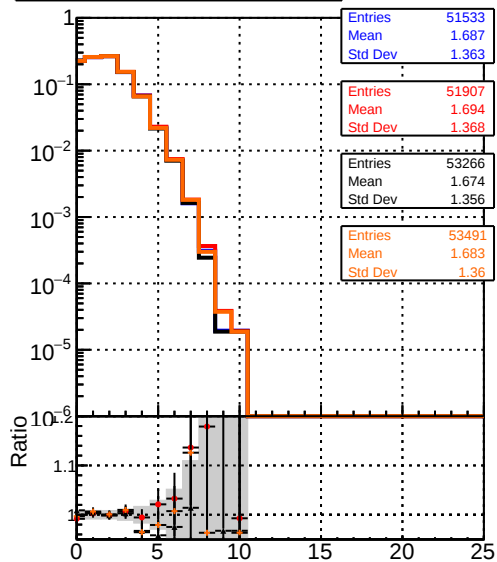
DQM_mkFit6_TT_base DQM_mkFit5_TT_retrainOldFiles125_v2_prelimWP_epoch4 DQM_mkFit6_TT_baseline_6iter DQM_mkFit6_TT_retrainOldFiles125_v2_prelimWP_epoch4
