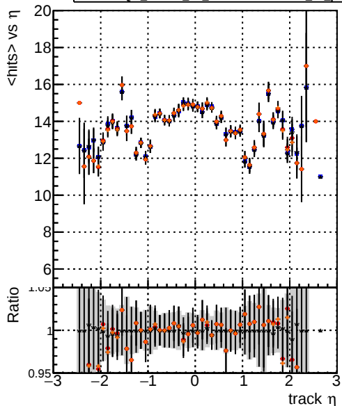
mean hits vs \eta DQM_mkFit1_TTbase DQM_mkFit5_TT_retrainOldFiles125_v2_prelimWP_epoch4 DQM_mkFit6_TT_baseline_6iter DQM_mkFit6_TT_retrainOldFiles125_v2_prelimWP_epoch4
