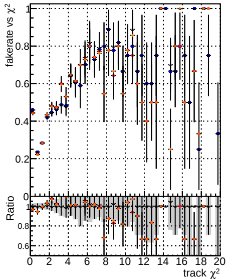
Fake rate vs. \chi^2 Legend: DQM mkFit TTbase, DQM mkFit TTbase, DQM mkFit TTbase
