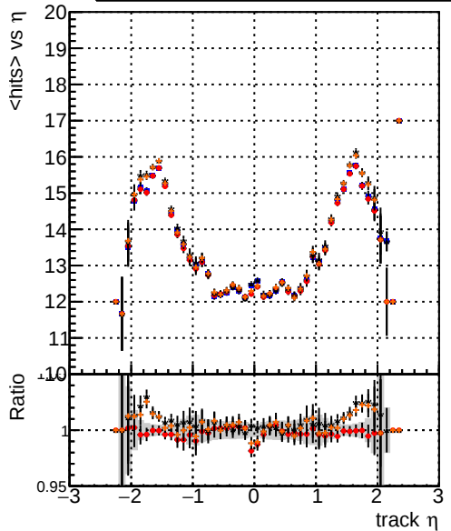
DQM_mkFit_TT_base DQM_mkFit5_TT_retrainOldFiles125_v2_prelimWP_epoch4 DQM_mkFit_TT_baseline_6iter DQM_mkFit6_TT_retrainOldFiles125_v2_prelimWP_epoch4
