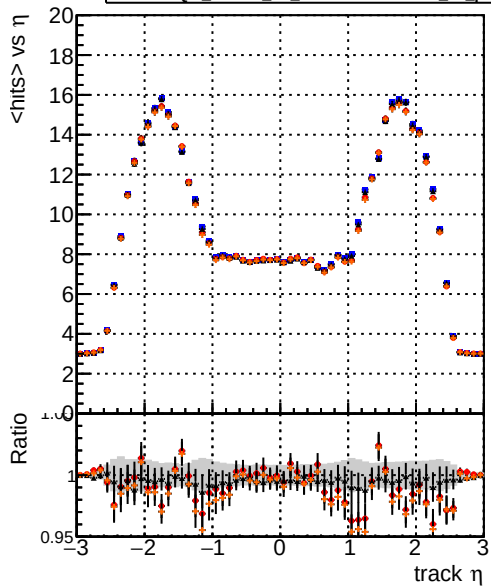
mean hit DQM_mkFit1_TTbase DQM_mkFit5_TT_retrainOldFiles125_v2_prelimWP_epoch4 DQM_mkFit6_TT_retrainOldFiles125_v2_prelimWP_epoch4
