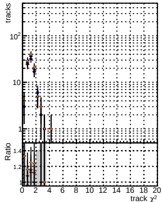
N of reco track vs. \chi^2 for BSM mFit TTbase, BSM mFit TTbase + L1, BSM mFit TTbase + L1 + L2, BSM mFit TTbase + L1 + L2 + L3, BSM mFit TTbase + L1 + L2 + L3 + L4, BSM mFit TTbase + L1 + L2 + L3 + L4 + L5, BSM mFit TTbase + L1 + L2 + L3 + L4 + L5 + L6, BSM mFit TTbase + L1 + L2 + L3 + L4 + L5 + L6 + L7, BSM mFit TTbase + L1 + L2 + L3 + L4 + L5 + L6 + L7 + L8, BSM mFit TTbase + L1 + L2 + L3 + L4 + L5 + L6 + L7 + L8 + L9, BSM mFit TTbase + L1 + L2 + L3 + L4 + L5 + L6 + L7 + L8 + L9 + L10, BSM mFit TTbase + L1 + L2 + L3 + L4 + L5 + L6 + L7 + L8 + L9 + L10 + L11, BSM mFit TTbase + L1 + L2 + L3 + L4 + L5 + L6 + L7 + L8 + L9 + L10 + L11 + L12, BSM mFit TTbase + L1 + L2 + L3 + L4 + L5 + L6 + L7 + L8 + L9 + L10 + L11 + L12 + L13, BSM mFit TTbase + L1 + L2 + L3 + L4 + L5 + L6 + L7 + L8 + L9 + L10 + L11 + L12 + L13 + L14, BSM mFit TTbase + L1 + L2 + L3 + L4 + L5 + L6 + L7 + L8 + L9 + L10 + L11 + L12 + L13 + L14 + L15, BSM mFit TTbase + L1 + L2 + L3 + L4 + L5 + L6 + L7 + L8 + L9 + L10 + L11 + L12 + L13 + L14 + L15 + L16, BSM mFit TTbase + L1 + L2 + L3 + L4 + L5 + L6 + L7 + L8 + L9 + L10 + L11 + L12 + L13 + L14 + L15 + L16 + L17, BSM mFit TTbase + L1 + L2 + L3 + L4 + L5 + L6 + L7 + L8 + L9 + L10 + L11 + L12 + L13 + L14 + L15 + L16 + L17 + L18, BSM mFit TTbase + L1 + L2 + L3 + L4 + L5 + L6 + L7 + L8 + L9 + L10 + L11 + L12 + L13 + L14 + L15 + L16 + L17 + L18 + L19, BSM mFit TTbase + L1 + L2 + L3 + L4 + L5 + L6 + L7 + L8 + L9 + L10 + L11 + L12 + L13 + L14 + L15 + L16 + L17 + L18 + L19 + L20
