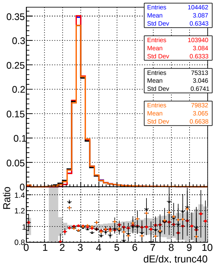
— DQM_mkFit_TTbase — DQM_mkFit5_TT_retrainOldFiles125_v2_prelimWP_epoch4 — DQM_mkFit_TT_baseline_6iter — DQM_mkFit6_TT_retrainOldFiles125_v2_prelimWP_epoch4
