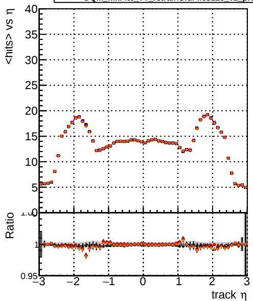
mean hits vs \eta DQM_mkFit_TTbase DQM_mkFit5_TT_retrainOldFiles125_v2_prelimWP_epoch4 DQM_mkFit_TT_baseline_6iter DQM_mkFit6_TT_retrainOldFiles125_v2_prelimWP_epoch4
