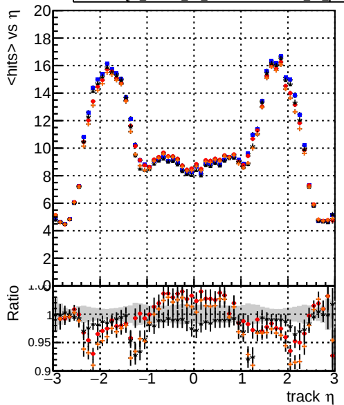
mean hit — DQM_mkFit6_TT_base — DQM_mkFit5_TT_retrainOldFiles125_v2_prelimWP_epoch4 — DQM_mkFit6_TT_retrainOldFiles125_v2_prelimWP_epoch4
