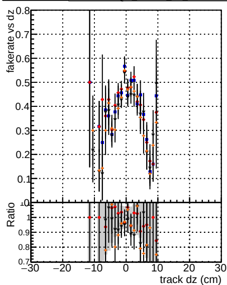
Fake rate vs dz Legend: DGM mkFit TTbase DGM mkFit TTbase DGM mkFit TTbase
