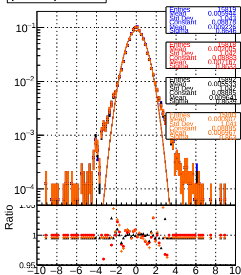
V2 preIMWP epoch4 pull of \theta parameter
