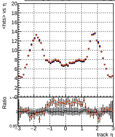
DQM_mkFit_TTbase DQM_mkFit5_TT_retrainOldFiles125_v2_prelimWP_epoch4 DQM_mkFit_TT_baseline_6iter DQM_mkFit6_TT_retrainOldFiles125_v2_prelimWP_epoch4 mean hits
