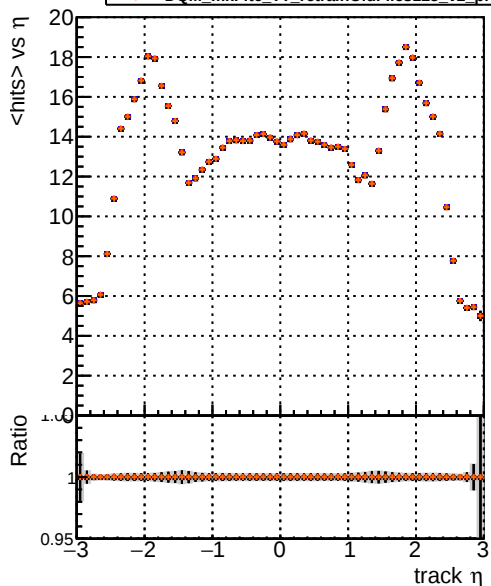
— DQM_mkFit_TTbase — DQM_mkFit5_TT_retrainOldFiles125_v2_prelimWP_epoch4 — DQM_mkFit6_TT_retrainOldFiles125_v2_prelimWP_epoch4 mean hits
