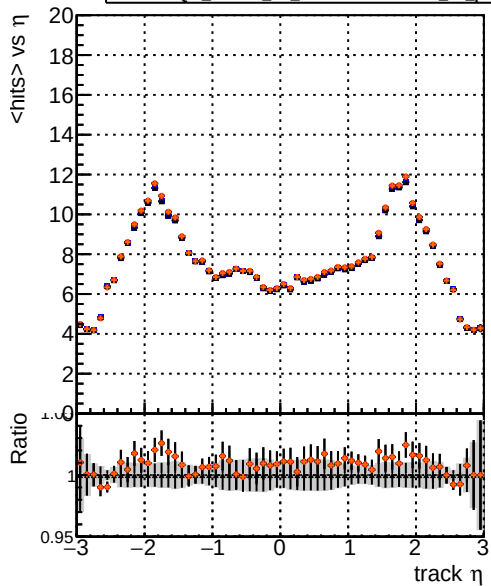
mean hits vs \eta DQM_mkFit TTbase DQM_mkFit5 TT_retrainOldFiles125_v2_prelimWP_epoch4 DQM_mkFit TT_baseline_6iter DQM_mkFit6 TT_retrainOldFiles125_v2_prelimWP_epoch4
