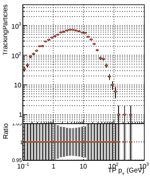
◆ DQM_mkFit6_TTbase ◆ DQM_mkFit5_TT_retrainOldFiles125_v2_prelimWP_epoch4 ◆ DQM_mkFit6_TT_retrainOldFiles125_v2_prelimWP_epoch4 ◆ DQM_mkFit5_TT_baseLine_6iter
