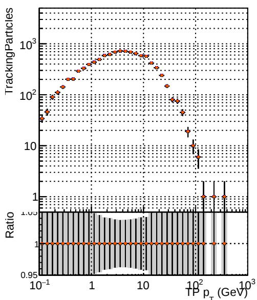
—•— DQM_mkFit6_TTbase —•— DQM_mkFit5_TT_retrainOldFiles125_v2_prelimWP_epoch4 —•— DQM_mkFit6_TT_retrainOldFiles125_v2_prelimWP_epoch4 —•— DQM_mkFit6_TT_baseLine_6iter
