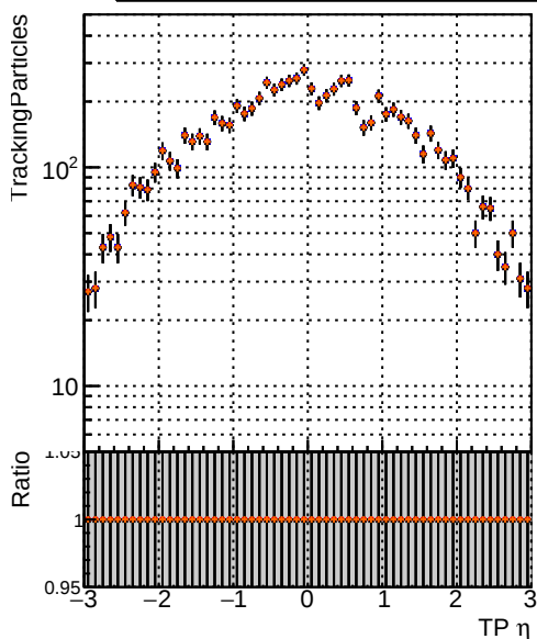
—•— DQM_mkFit6_TTbase —•— DQM_mkFit5_TT_retrainOldFiles125_v2_prelimWP_epoch4 —•— DQM_mkFit6_TT_retrainOldFiles125_v2_prelimWP_epoch4 —•— DQM_mkFit6_TT_baseLine_6iter
