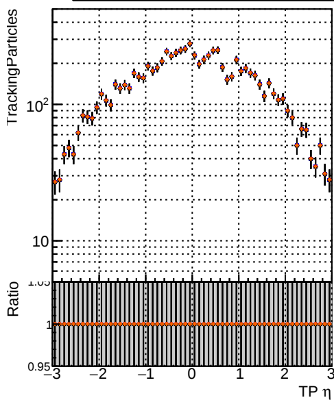
— DQM_mkFit6_TT_base — DQM_mkFit5_TT_retrainOldFiles125_v2_prelimWP_epoch4 — DQM_mkFit6_TT_base — DQM_mkFit6_TT_retrainOldFiles125_v2_prelimWP_epoch4
