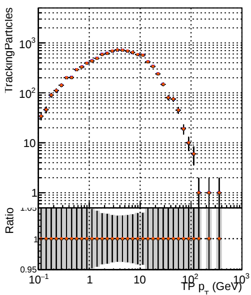
—•— DQM_mkFit6_TTbase —•— DQM_mkFit5_TT_retrainOldFiles125_v2_prelimWP_epoch4 —•— DQM_mkFit6_TT_baseLine_6iter —•— DQM_mkFit6_TT_retrainOldFiles125_v2_prelimWP_epoch4
