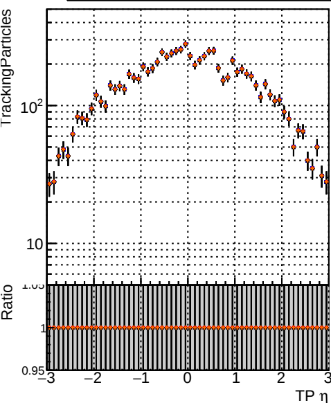
—•— DQM_mkFit6_TTbase —•— DQM_mkFit5_TT_retrainOldFiles125_v2_prelimWP_epoch4 —•— DQM_mkFit6_TT_baseLine_6iter —•— DQM_mkFit6_TT_retrainOldFiles125_v2_prelimWP_epoch4
