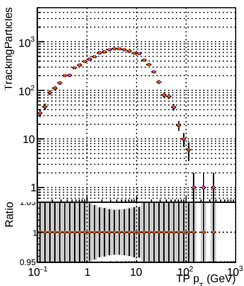
— DQM_mkFit6_TT_retrainOldFiles125_v2_prelimWP_epoch4 — DQM_mkFit5_TT_retrainOldFiles125_v2_prelimWP_epoch4 — DQM_mkFit6_TT_retrainOldFiles125_v2_prelimWP_epoch4 — DQM_mkFit5_TT_retrainOldFiles125_v2_prelimWP_epoch4
