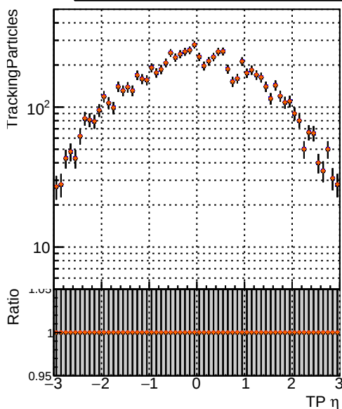
— DQM_mkFit6_TT_retrainOldFiles125_v2_prelimWP_epoch4 — DQM_mkFit5_TT_retrainOldFiles125_v2_prelimWP_epoch4 — DQM_mkFit6_TT_retrainOldFiles125_v2_prelimWP_epoch4 — DQM_mkFit5_TT_retrainOldFiles125_v2_prelimWP_epoch4
