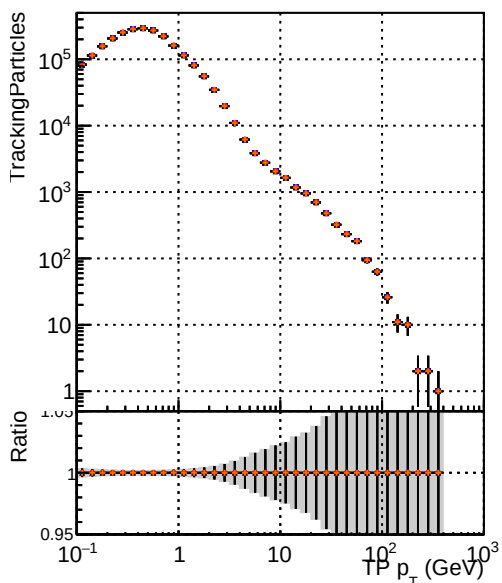
—●— DQM_mkFit6_TTbase —●— DQM_mkFit5_TT_retrainOldFiles125_v2_prelimWP_epoch4 —●— DQM_mkFit6_TT_retrainOldFiles125_v2_prelimWP_epoch4 —●— DQM_mkFit6_TT_base6iter
