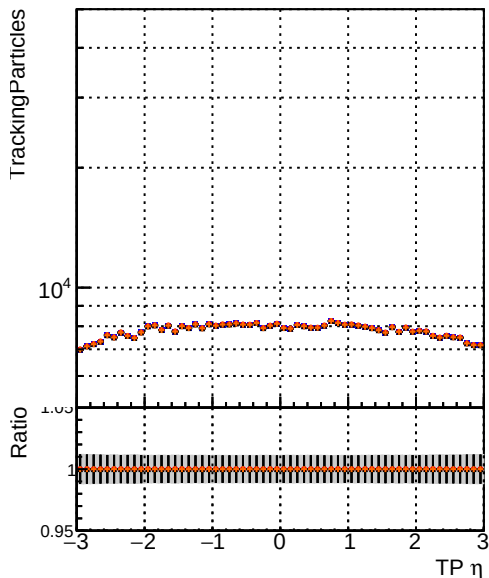
—●— DQM_mkFit6_TTbase —●— DQM_mkFit5_TT_retrainOldFiles125_v2_prelimWP_epoch4 —●— DQM_mkFit6_TT_retrainOldFiles125_v2_prelimWP_epoch4 —●— DQM_mkFit6_TT_base6iter
