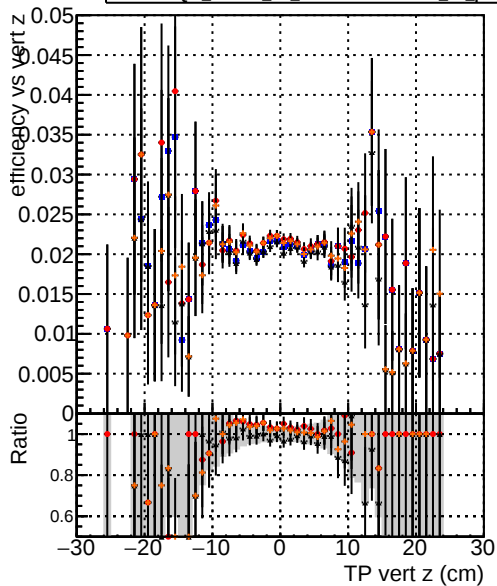
Efficiency vs vert z —●— DQM_mkFit1_TTbase —●— DQM_mkFit5_TT_retrainOldFiles125_v2_prelimWP_epoch4 —●— DQM_mkFit6_TT_retrainOldFiles125_v2_prelimWP_epoch4 —●— DQM_mkFit_TT_baseline_6iter
