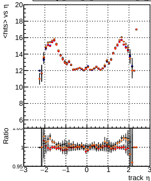
mean hits DQM_mkFit6_TT_base DQM_mkFit5_TT_retrainOldFiles125_v2_prelimWP_epoch4 DQM_mkFit6_TT_base DQM_mkFit6_TT_retrainOldFiles125_v2_prelimWP_epoch4
