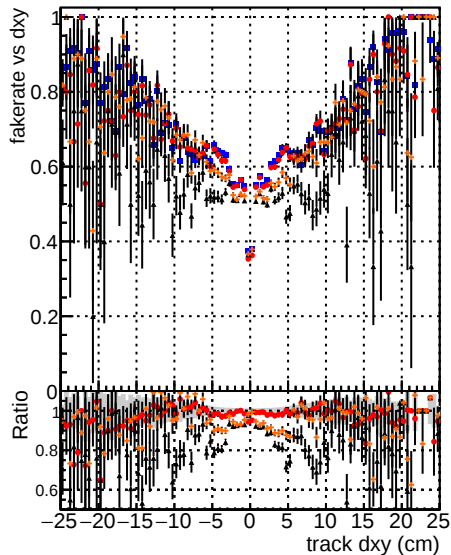
Fake rate vs d DGM mkFit TTbase DGM mkFit TTbase DGM mkFit TTbase DGM mkFit TTbase
