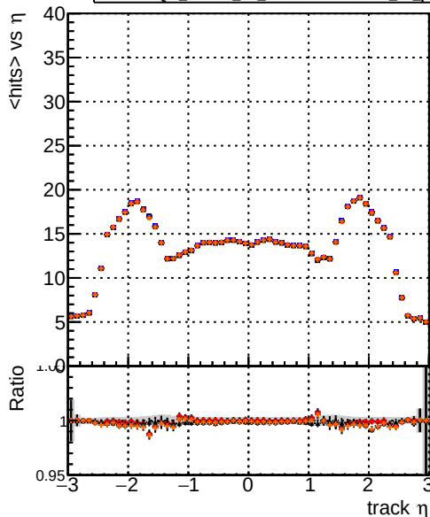
mean hits DQM_mkFit6 TT_base DQM_mkFit5 TT_retrainOldFiles125_v2_prelimWP_epoch4 DQM_mkFit6 TT_retrainOldFiles125_v2_prelimWP_epoch4 DQM_mkFit6 TT_base
