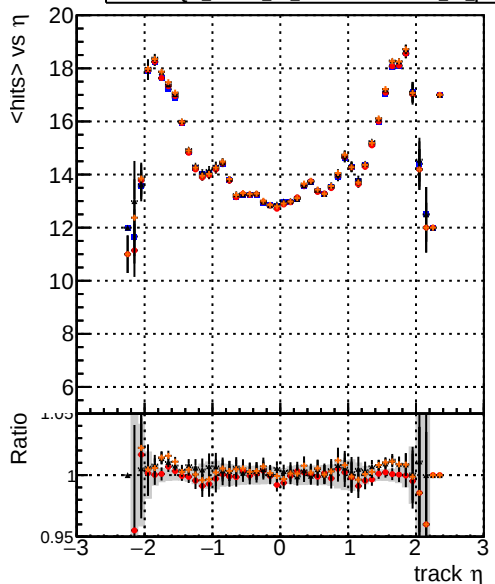
mean hit DQM_mkFit_TTbase DQM_mkFit5_TT_retrainOldFiles125_v2_prelimWP_epoch4 DQM_mkFit6_TT_retrainOldFiles125_v2_prelimWP_epoch4 DQM_mkFit_TT_baseLine_6iter
