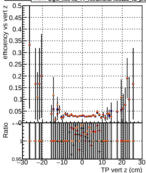
Efficiency vs vert z —•— DQM_mkFit1_TTbase —•— DQM_mkFit5_TT_retrainOldFiles125_v2_prelimWP_epoch4 —•— DQM_mkFit6_TT_retrainOldFiles125_v2_prelimWP_epoch4 —•— DQM_mkFit1_TTbase —•— DQM_mkFit5_TT_retrainOldFiles125_v2_prelimWP_epoch4 —•— DQM_mkFit6_TT_retrainOldFiles125_v2_prelimWP_epoch4
