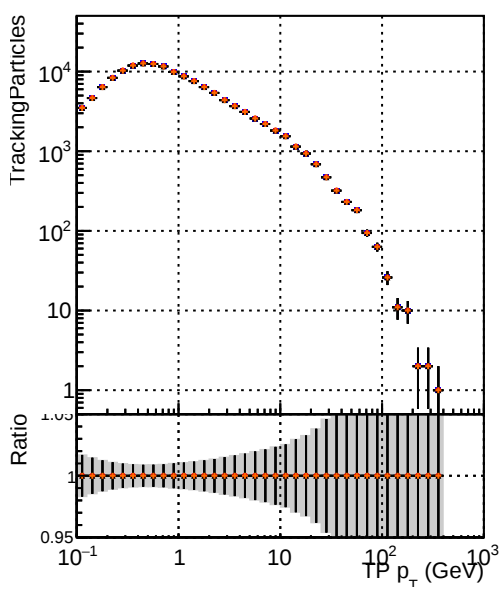
—●— DQM_mkFit1_TTbase —●— DQM_mkFit5_TT_retrainOldFiles125_v2_prelimWP_epoch4 —●— DQM_mkFit6_TT_retrainOldFiles125_v2_prelimWP_epoch4 —●— DQM_mkFit6_TT_retrainOldFiles125_v2_prelimWP_epoch4
