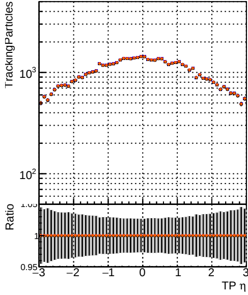
—●— DQM_mkFit1_TTbase —●— DQM_mkFit5_TT_retrainOldFiles125_v2_prelimWP_epoch4 —●— DQM_mkFit6_TT_retrainOldFiles125_v2_prelimWP_epoch4 —●— DQM_mkFit6_TT_retrainOldFiles125_v2_prelimWP_epoch4
