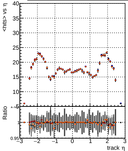
mean hits DQM_mkFit5_TT_retrainOldFiles125_v2_prelimWP_epoch4 DQM_mkFit6_TT_retrainOldFiles125_v2_prelimWP_epoch4 DQM_mkFit_TT_baseline_6iter
