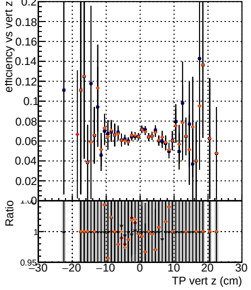
Efficiency vs. TP vert z (cm) —●— DQM_mkFit1_TTbase —◆— DQM_mkFit5_TT_retrainOldFiles125_v2_prelimWP_epoch4 —▲— DQM_mkFit_TT_baseline_6iter —△— DQM_mkFit6_TT_retrainOldFiles125_v2_prelimWP_epoch4
