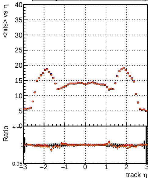
mean hits DQM_mkFit6_TT_base DQM_mkFit5_TT_retrainOldFiles125_v2_prelimWP_epoch4 DQM_mkFit6_TT_baseline_6iter DQM_mkFit6_TT_retrainOldFiles125_v2_prelimWP_epoch4
