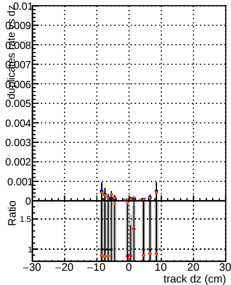
125_v2_prelimWP_epoch4
