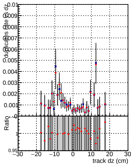
—●— DQM_CKF_XiMinusPU_base —●— DQM_CKF_XiMinusPU_retrainOldFiles125_v2_prelimWPM_epoch4
